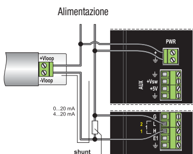
Trasmettitori con uscita in corrente a 2 fili
