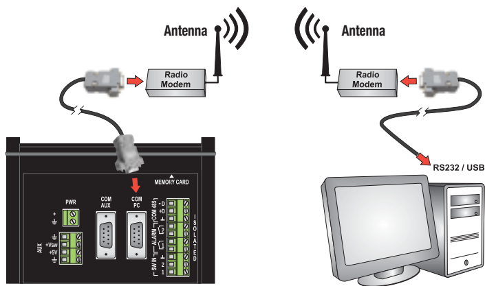
Comunicazione tramite Radio Modem VHF
