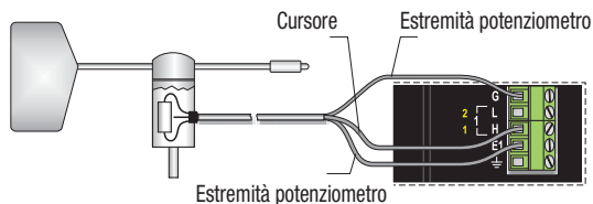
Sensori potenziometrici a 3 fili
