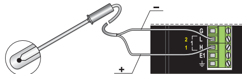
Termocoppie / sensori con uscita in mV
