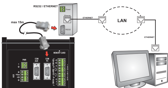
Comunicazione tramite rete locale con protocollo TCP/IP
