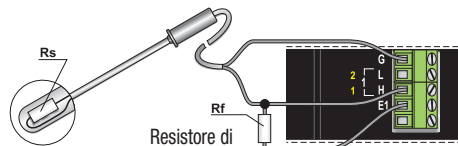
Sensori resistivi a 2 fili
