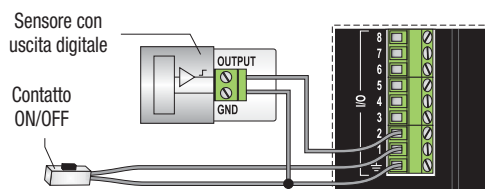
Rilevazione di stati logici
