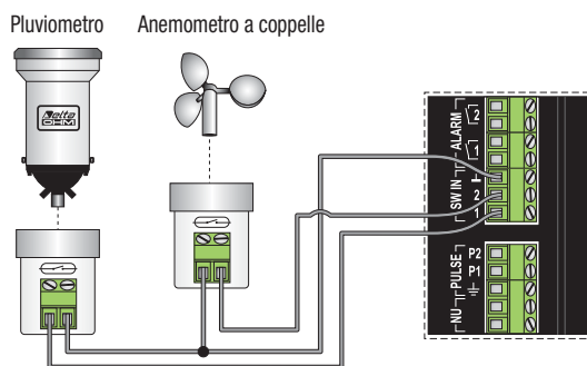
Sensori con uscita in frequenza a contatto
