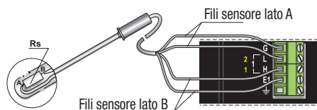
Sensori resistivi a 4 fili (Pt100/Pt1000)
