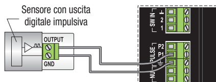
Sensori con uscita digitale in frequenza
