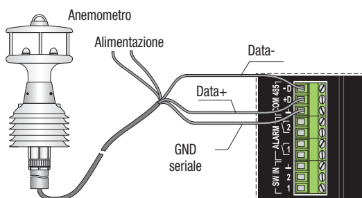
Anemometri Delta OHM Sensori con uscita RS485 Modbus-RTU
