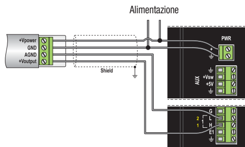
Trasmettitori con uscita in tensione
