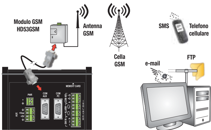
Comunicazione tramite rete GSM
